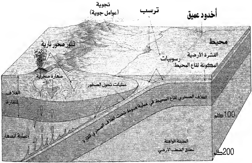
رسم تخطيطي لحركة الألواح الصخرية في قيعان المحيطات
